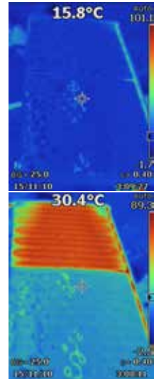
Prototype de capteur hybride associant les 2 technologies : standard (partie basse) et thermochrome (partie haute). Mise en évidence de l'effet thermochrome (augmentation du rayonnement thermique) à l'aide d'une caméra infrarouge.
